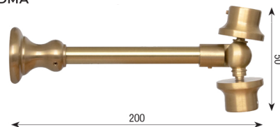
Mensola multiangolo ottone Ø14 Art. MS22MDMA
