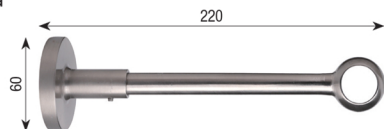
Mensola tonda singola chiusa Art. MS22MSC/T
