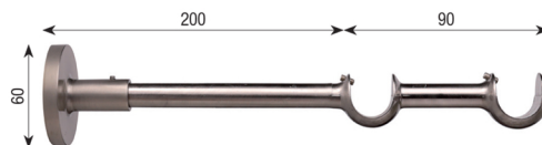
Mensola tonda doppia aperta Art. MS22MDA/T
