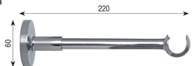
Mensola tonda singola aperta Art. MS22MSA/T
